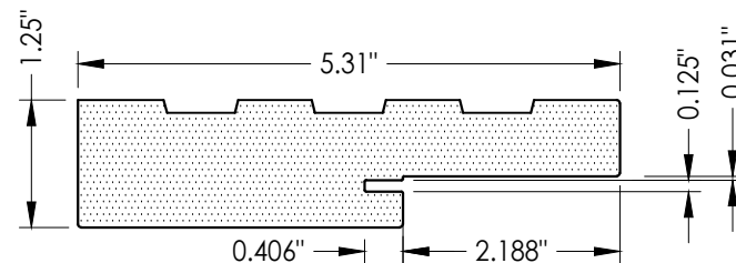
1 COMPOSITE JAMB
